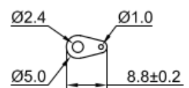
SOLDER LUG
