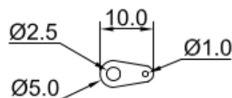
SOLDER LUG S=1:1
