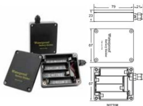
PBH-341-IP68-A
