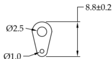
SOLDER LUG
