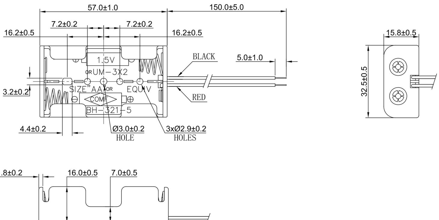
BH-321-5D Shown
