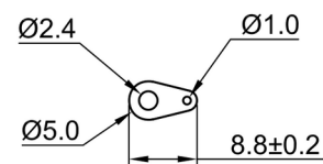
SOLDER LUG
